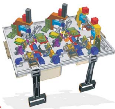
Varilna vpenjalna priprava za sklopko (3x2 gnezdi)
