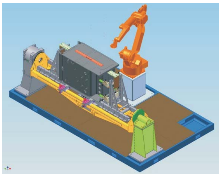
Razporeditev opreme varilne robotske celice
