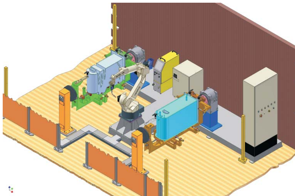
Razporeditev opreme varilne robotske celice
