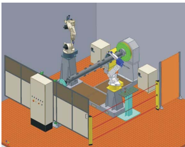
Razporeditev opreme varilne robotske celice
